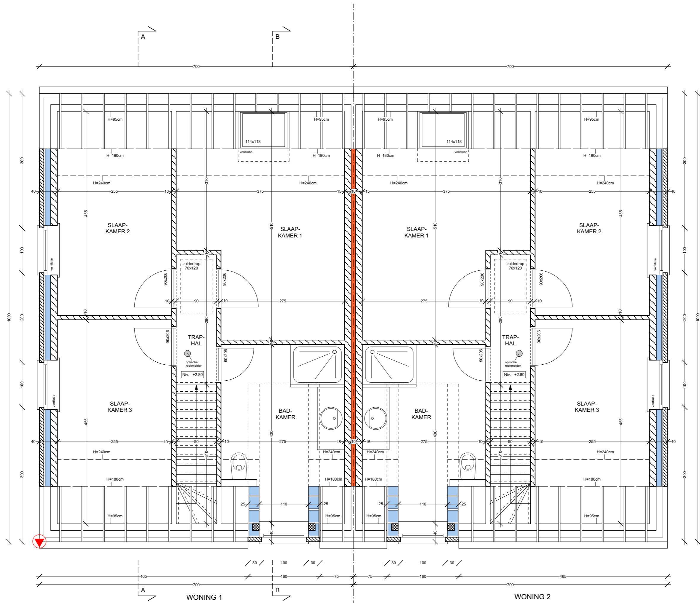
PLAN VERDIEPING schaal 1/50
